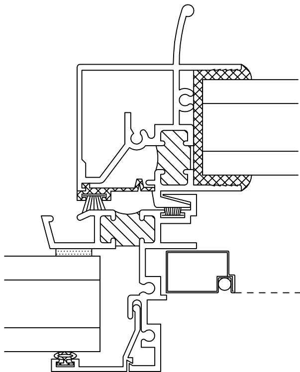
⑤ INTERLOCK
