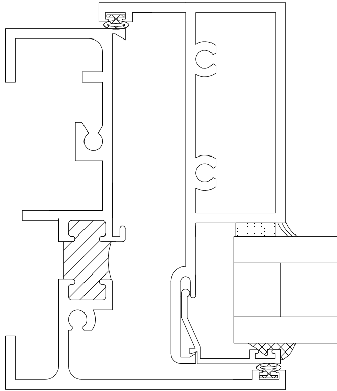
3 JAMB @ VENT
